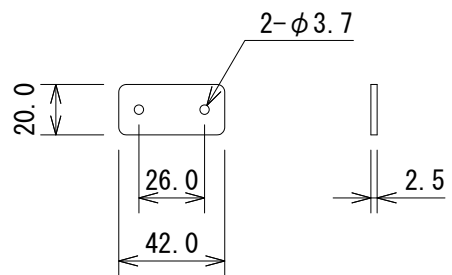
リンク金具
