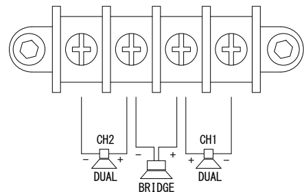
出力コネクター拡大図
