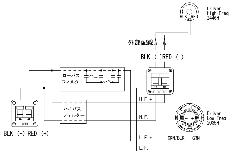
接続図
