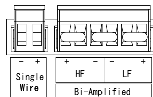
端子拡大図
