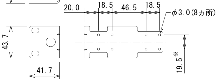
L字金具
