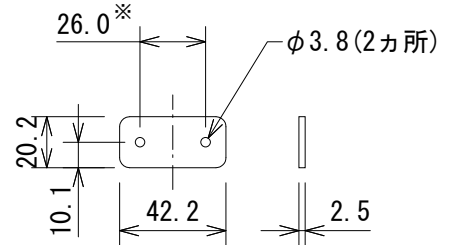
連結金具
