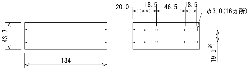
U字金具
