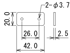
連結金具
