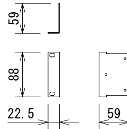
ラックマウント金具 (付属品)
