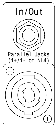
コネクターパネル拡大図
