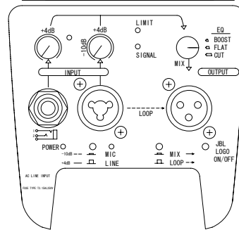
コネクターパネル拡大図
