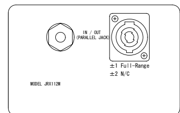
コネクターパネル拡大図
