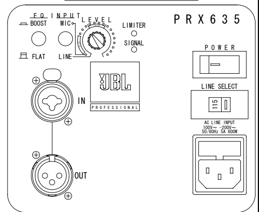
コネクターパネル拡大図
