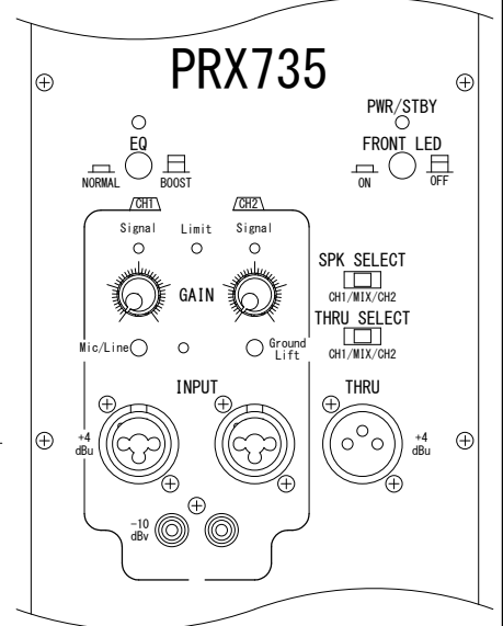
コネクターパネル拡大図
