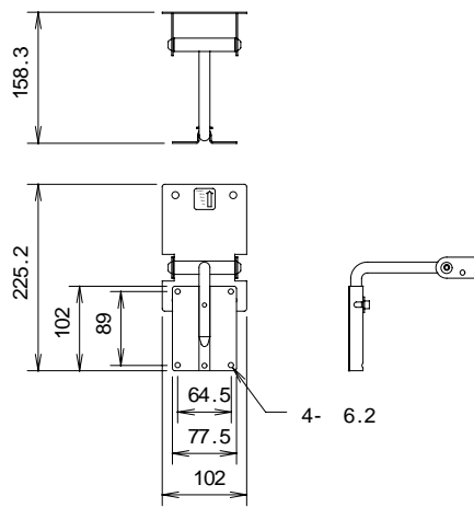
251取付金具
