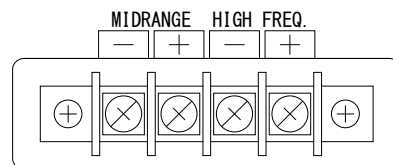
4732-M/HF-T (MF・HF) ネジ式ターミナル (4mm相当) 背面端子拡大図
