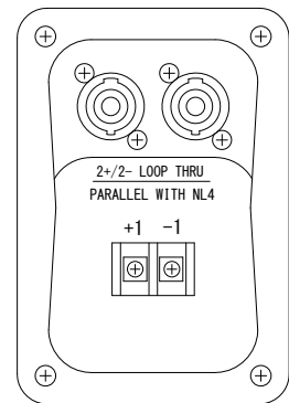
端子拡大図
