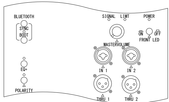
背面パネル拡大図
