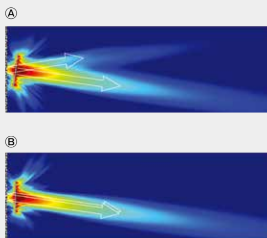
壁面に対して斜めに設置した通常のコラムスピーカー (A)と、垂直に設 置したIntellivox (B)。通常のコラムスピーカーでは、背面への放射音の 影響で斜め上に向かって意図しない音出力されてしまうが、Intellivoxは 背面への放射音の影響がほとんどなく、リスニングエリアに向けて出力パ ワーを集中できる。
