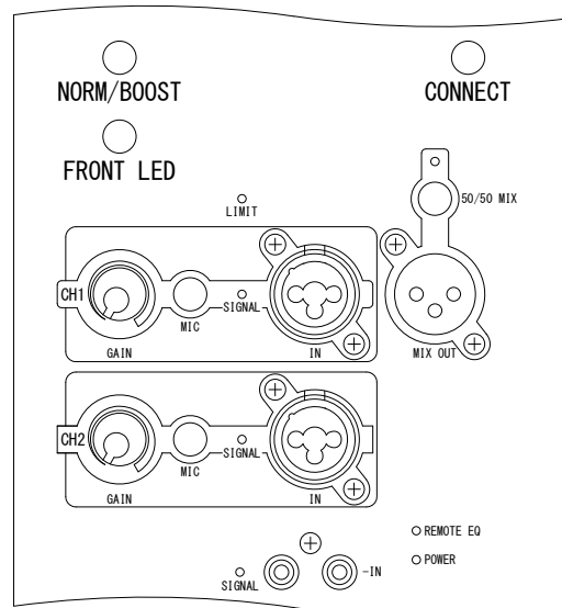
背面パネル拡大図
