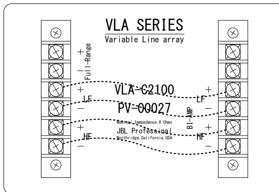
端子拡大図
