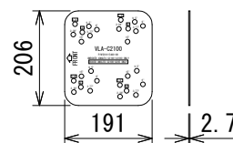
連結金具
