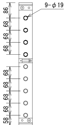
A-A''断面図
