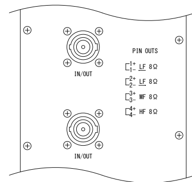
背面端子拡大図
