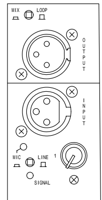
コネクターパネル拡大図
